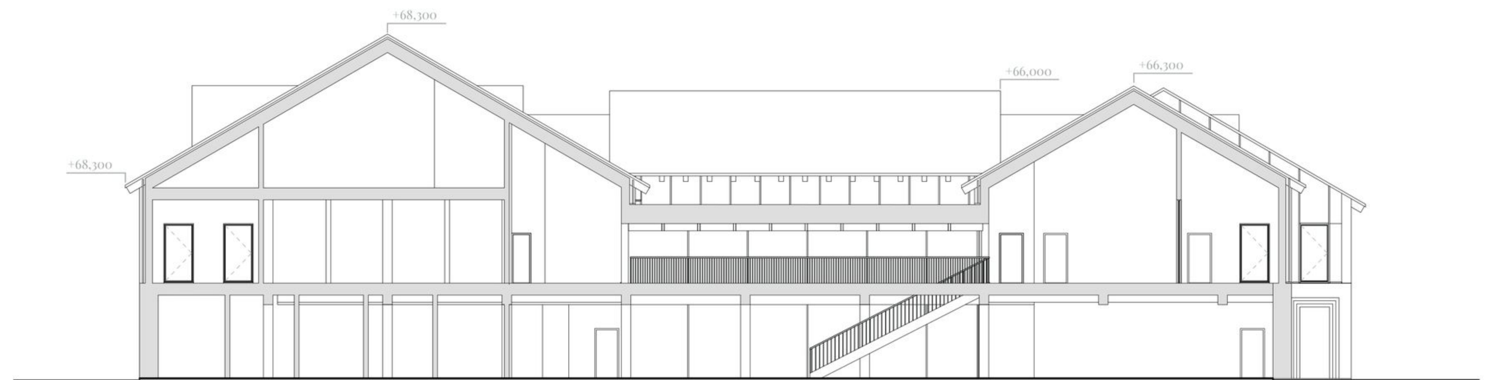
LEIKKAUS B-B / 1:250
