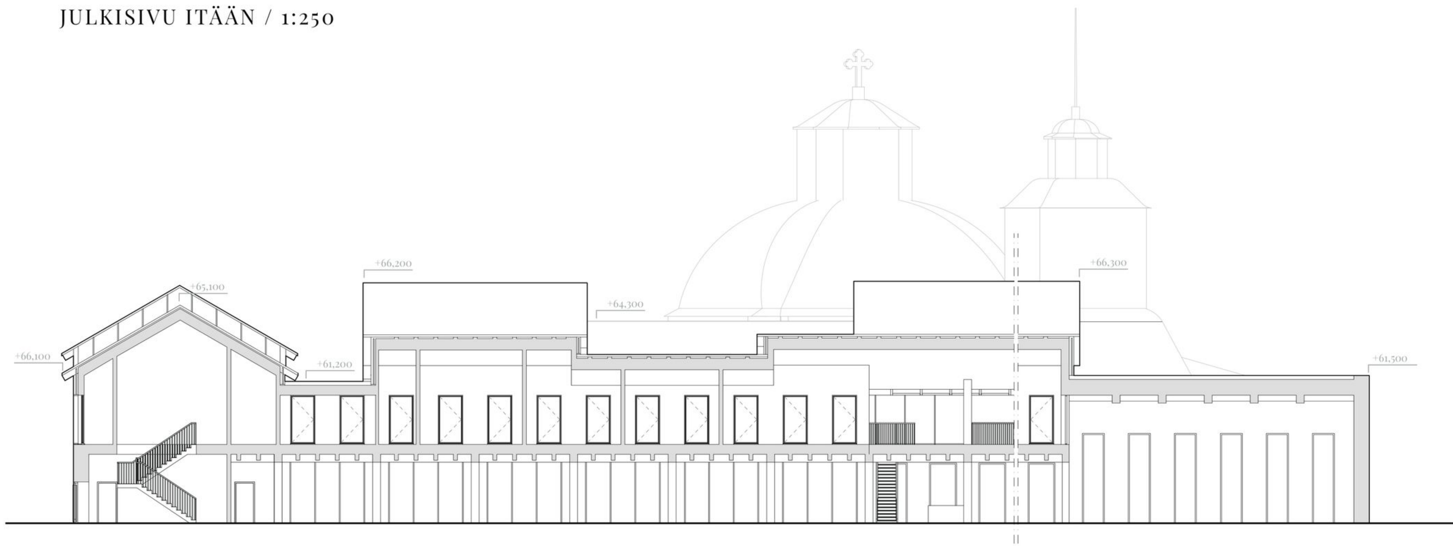
LEIKKAUS A-A / 1:250
