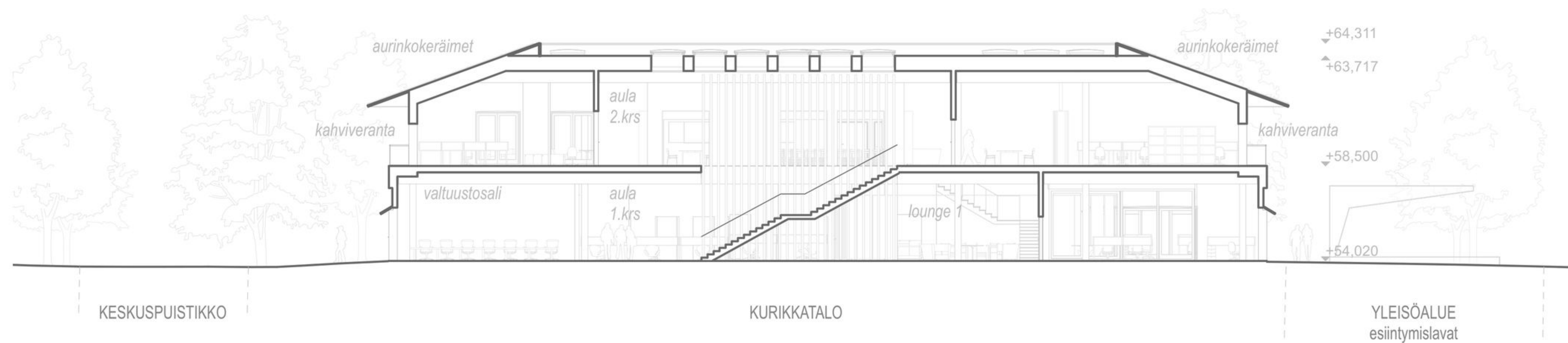
LEIKKAUS A-A 1:250
