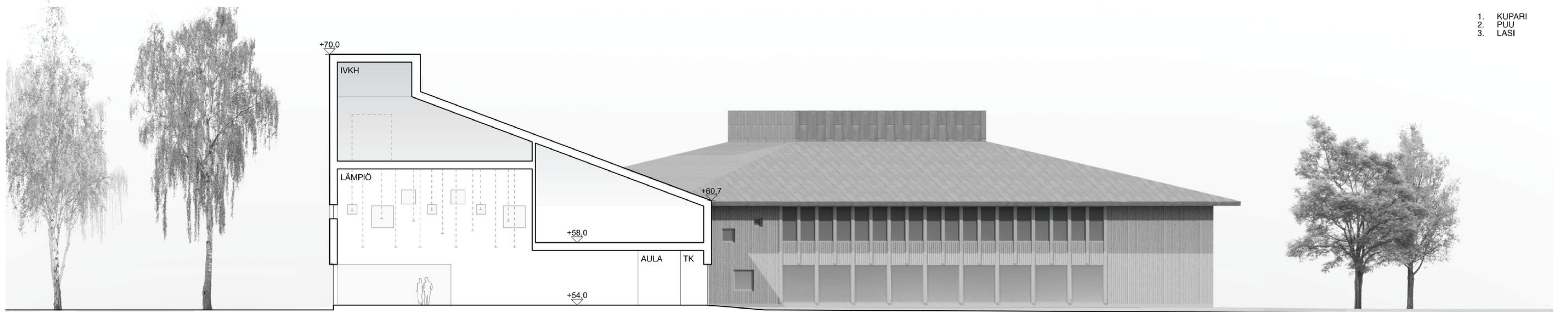
Leikkaus A-A 1:250
