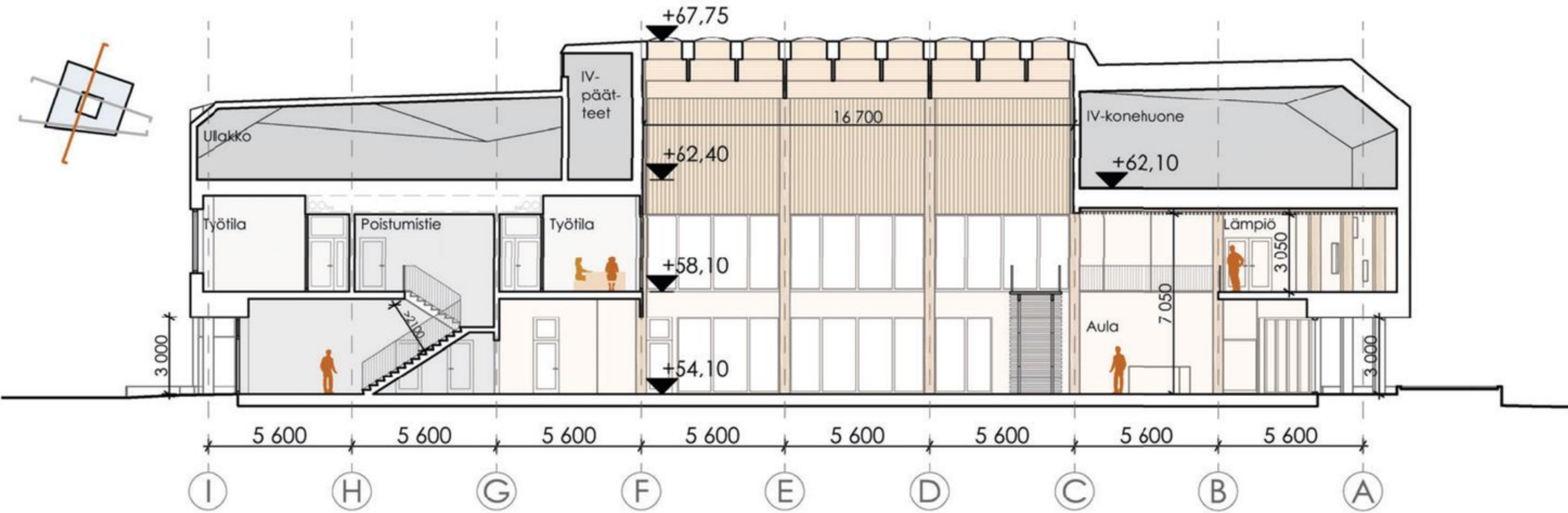
Leikkaus B-B' 1:300
