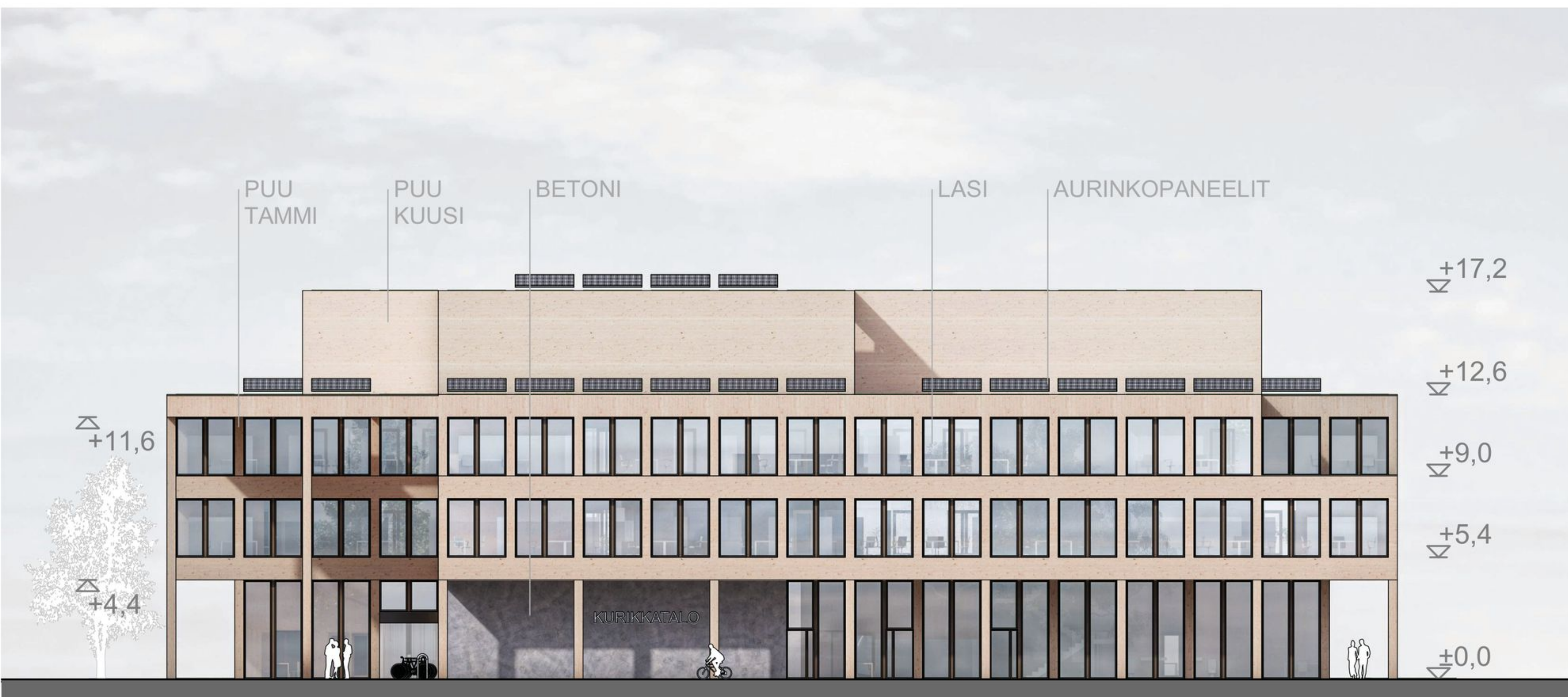
JULKISIVU ETELÄÄN 1:250
