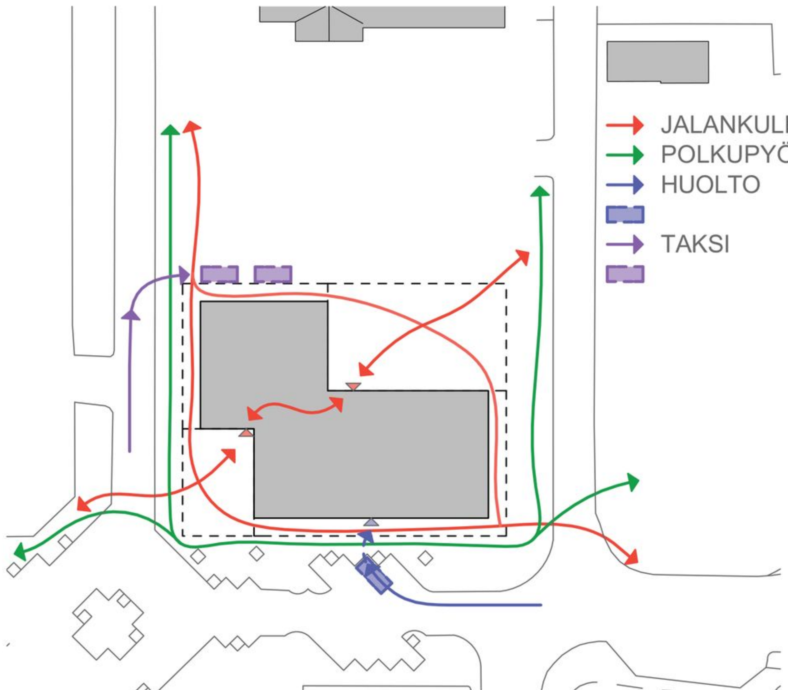
LIIKENNEKAAVIO
