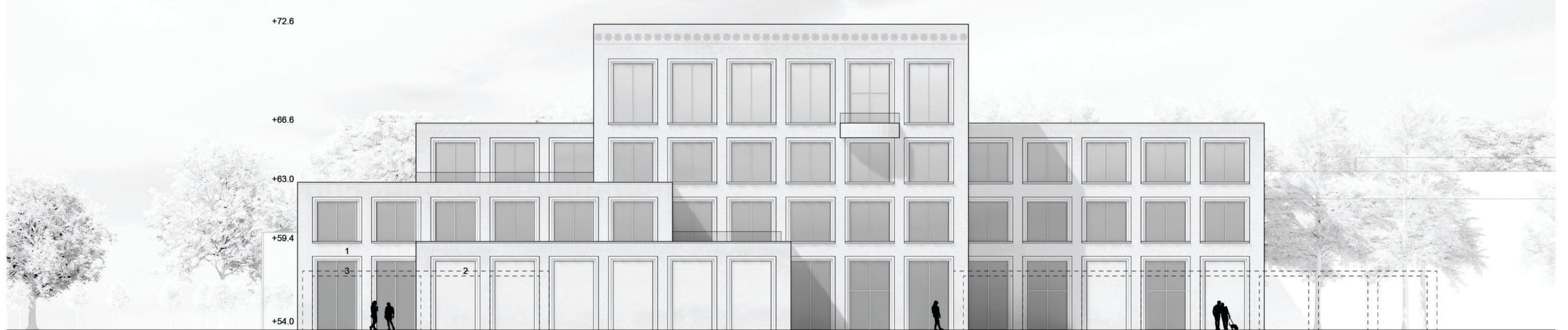
Julkisivu kaakkoon 1:250
