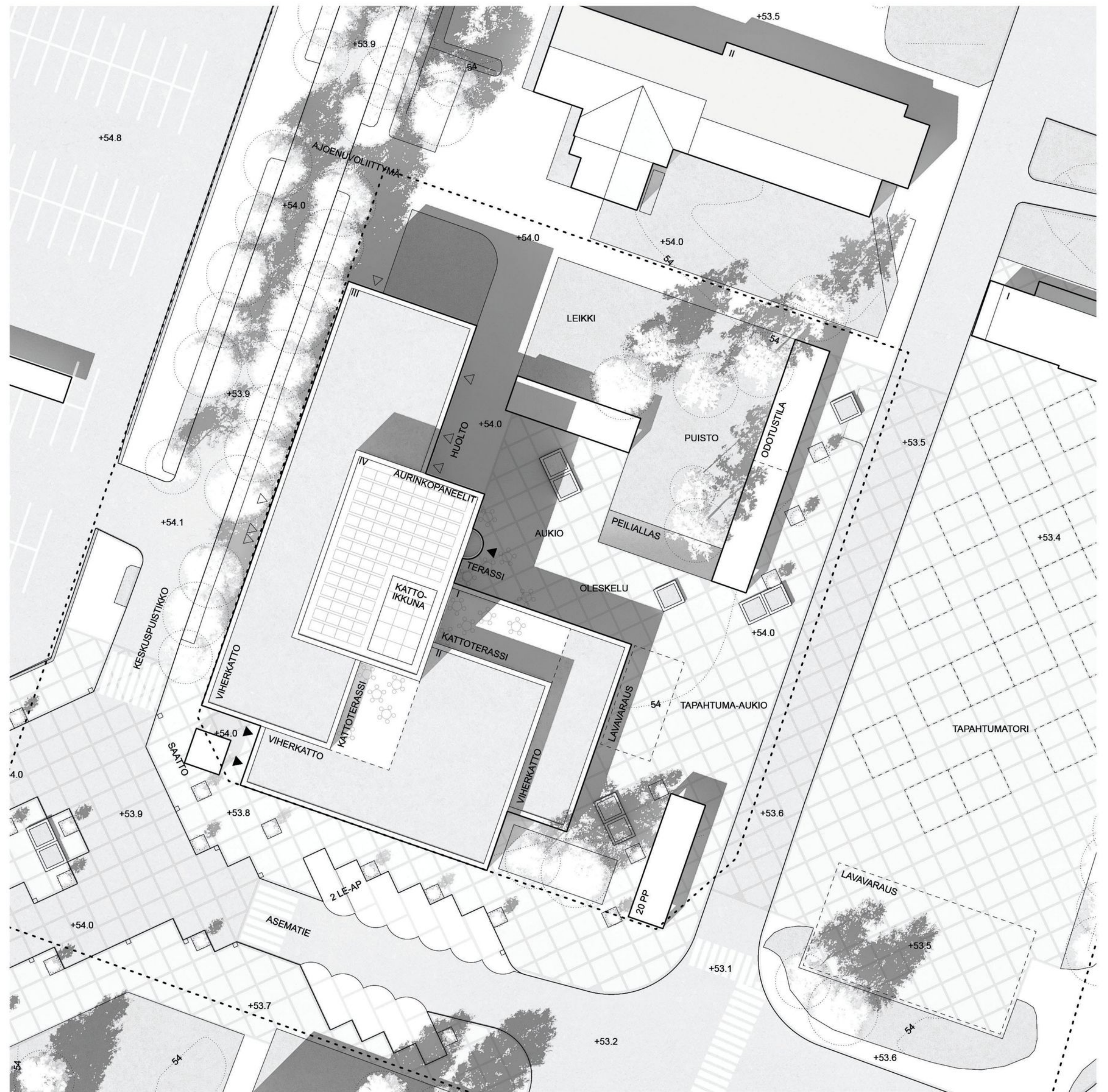
Asemapiirros 1:500
