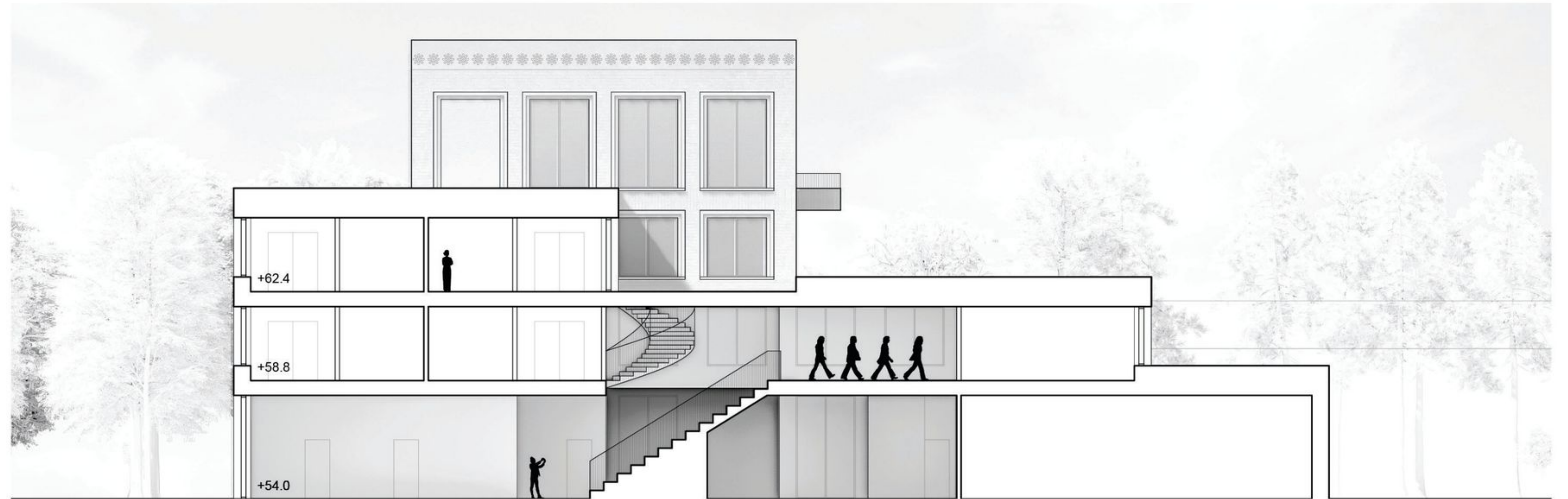
Leikkaus B-B 1:250
