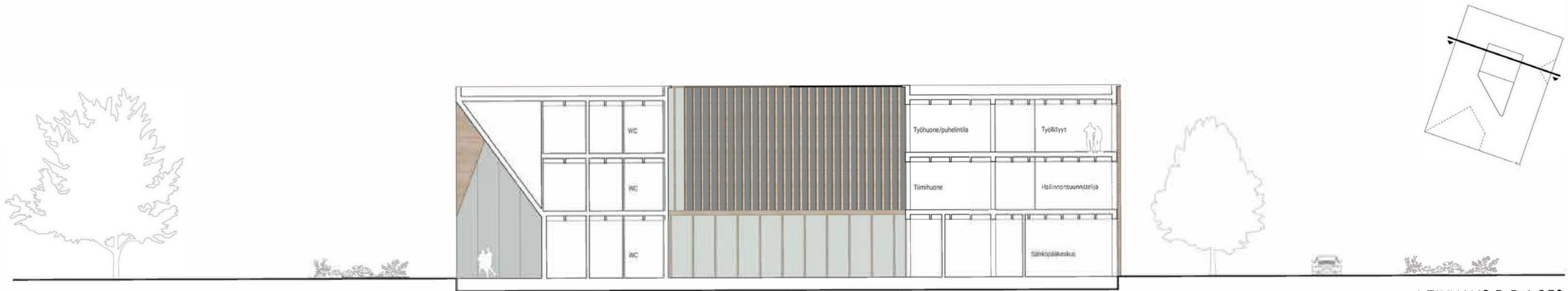
LEIKKAUS B-B 1:250
