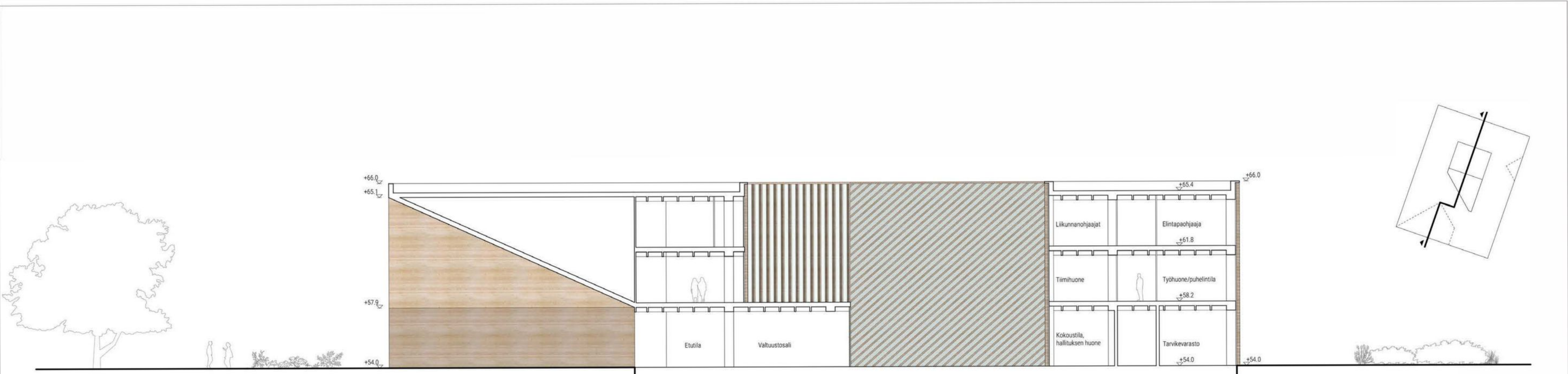
LEIKKAUS A-A 1:250
