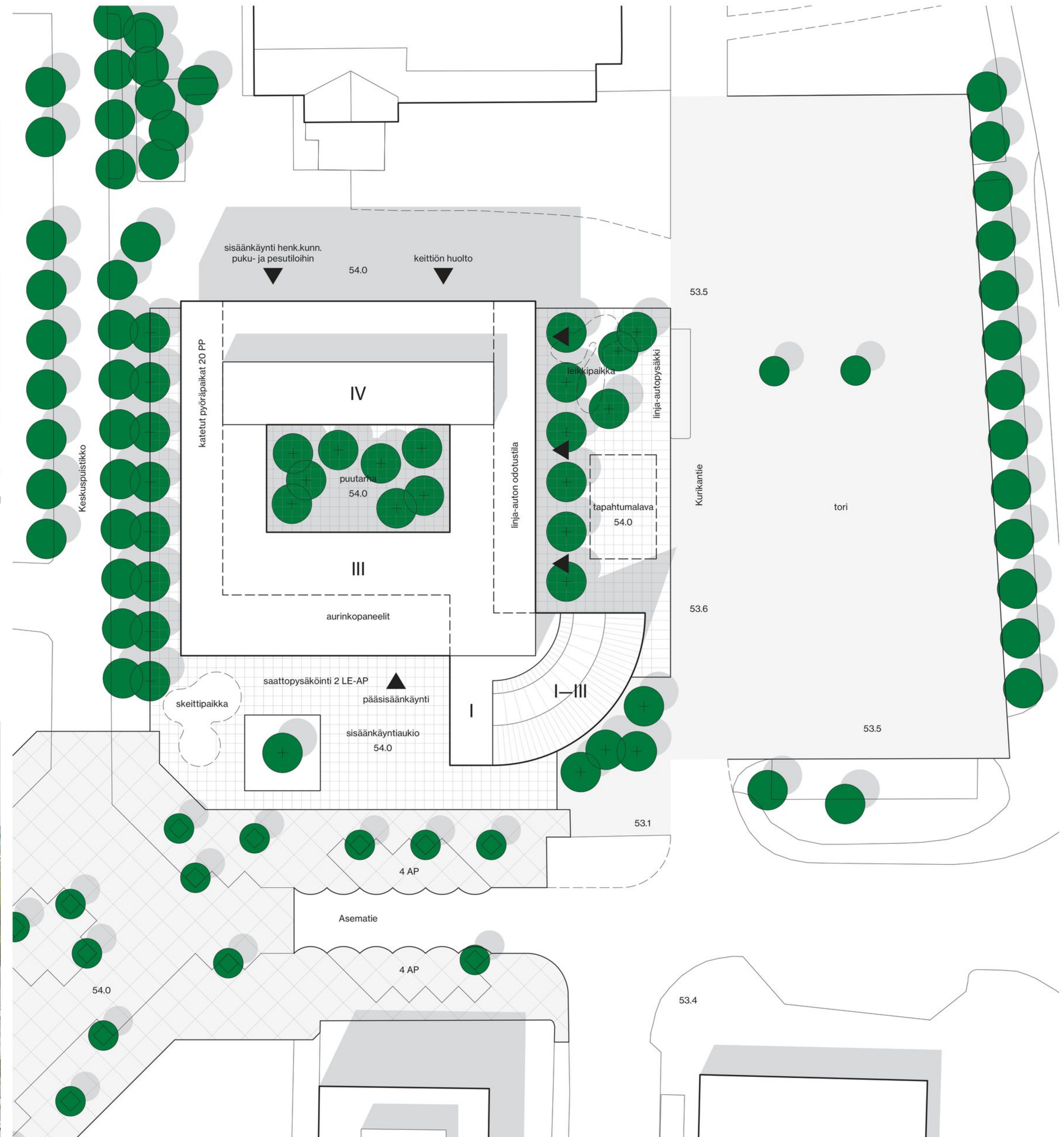
asemapiirros 1/500
