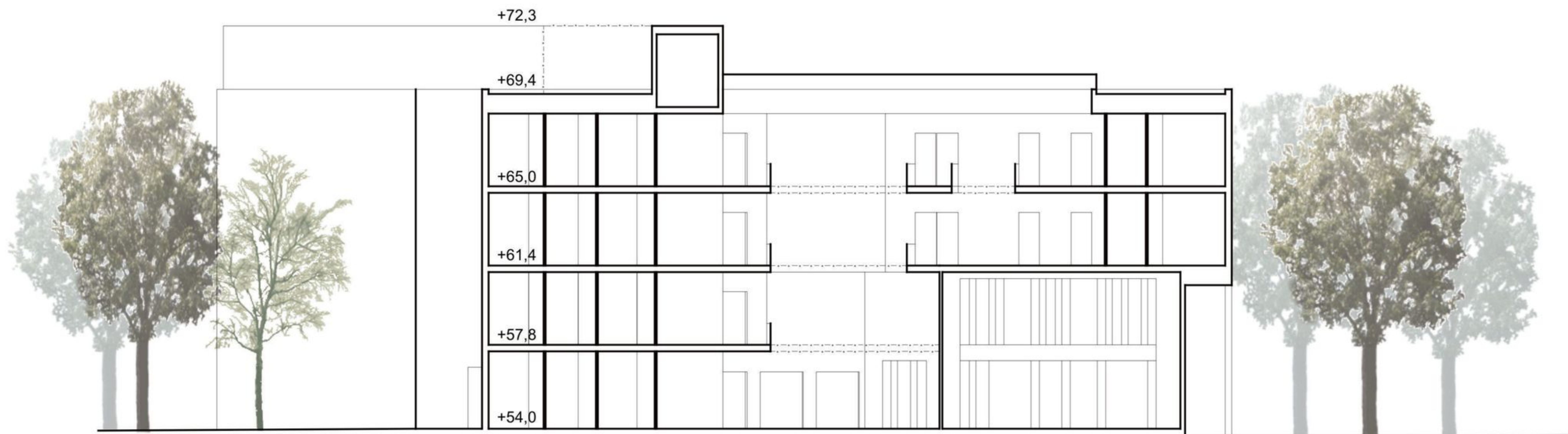
LEIKKAUS AA 1:250
