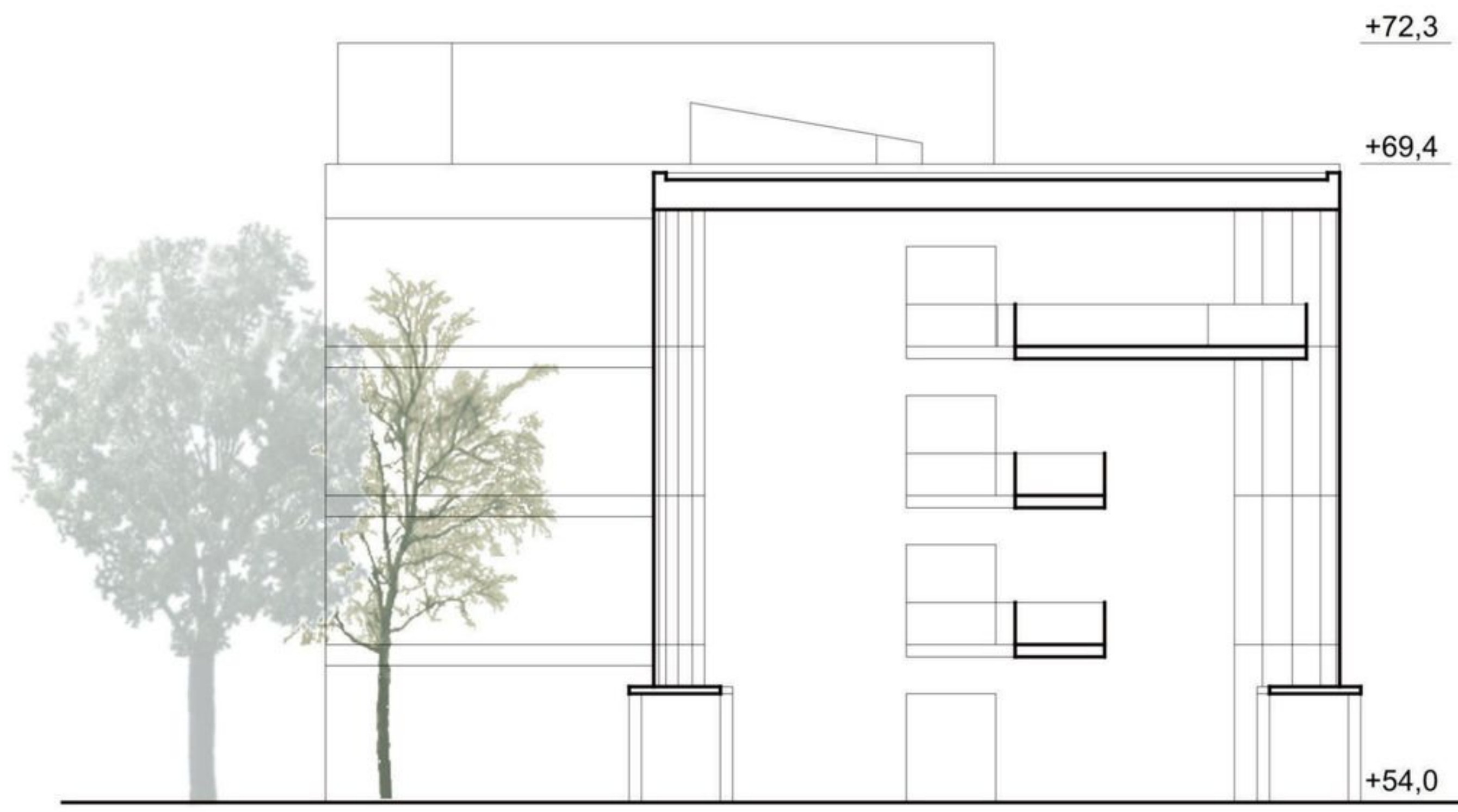
LEIKKAUS BB 1:250
