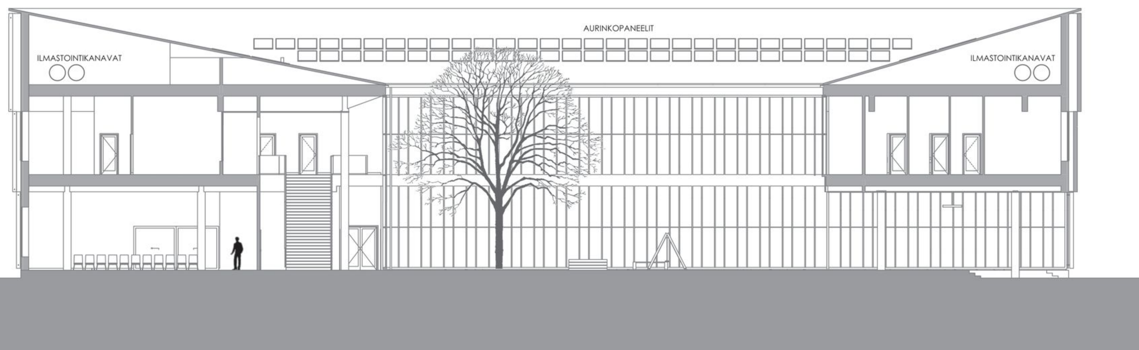
LEIKKAUS A-A
