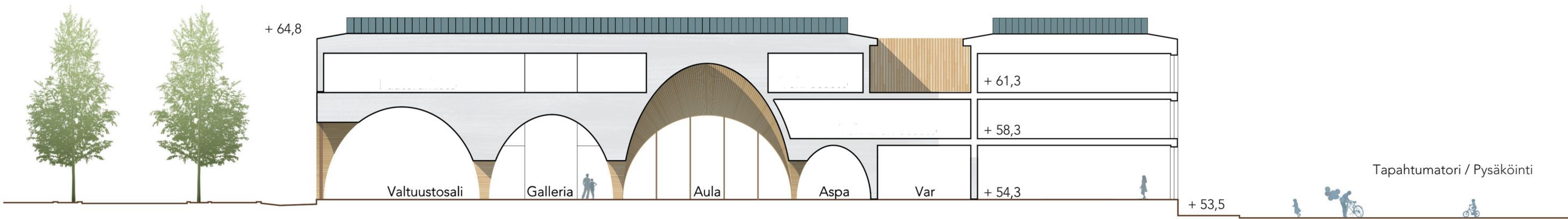
Leikkaus B 1:250
