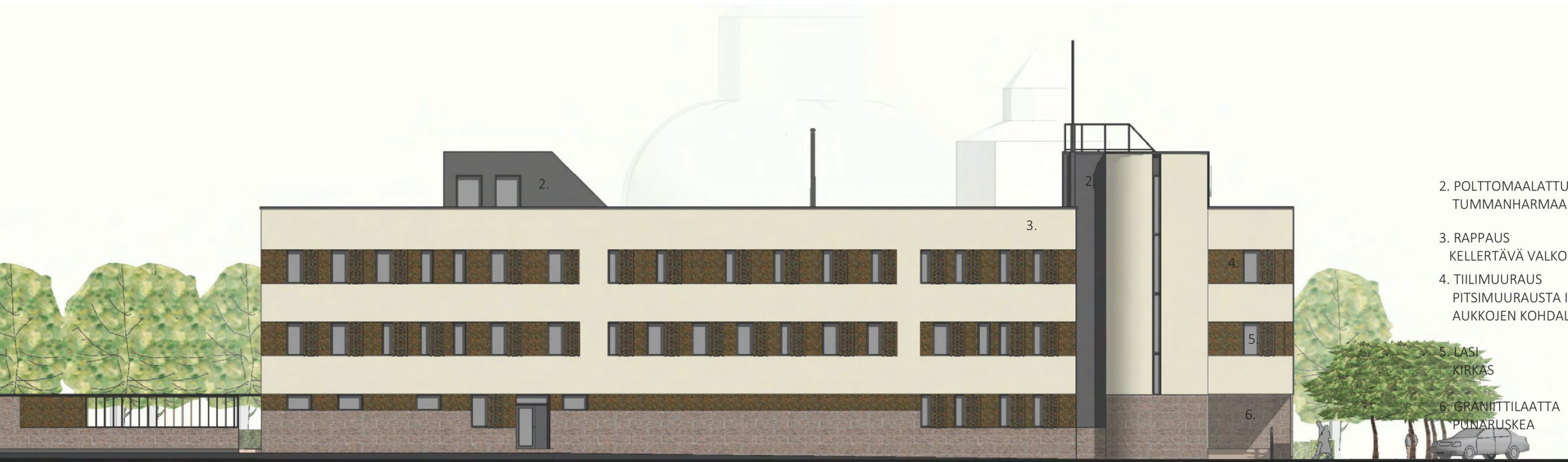
JULKISIVU LÄNTEEN 1:250
