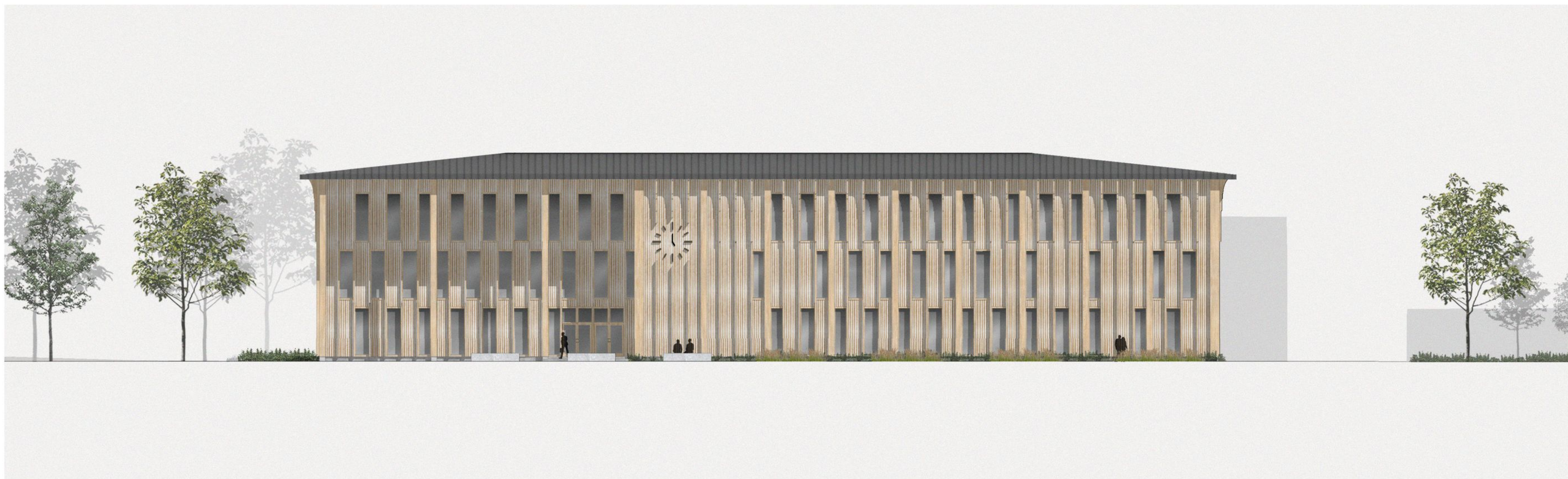
Julkisivu etelään 1:250
