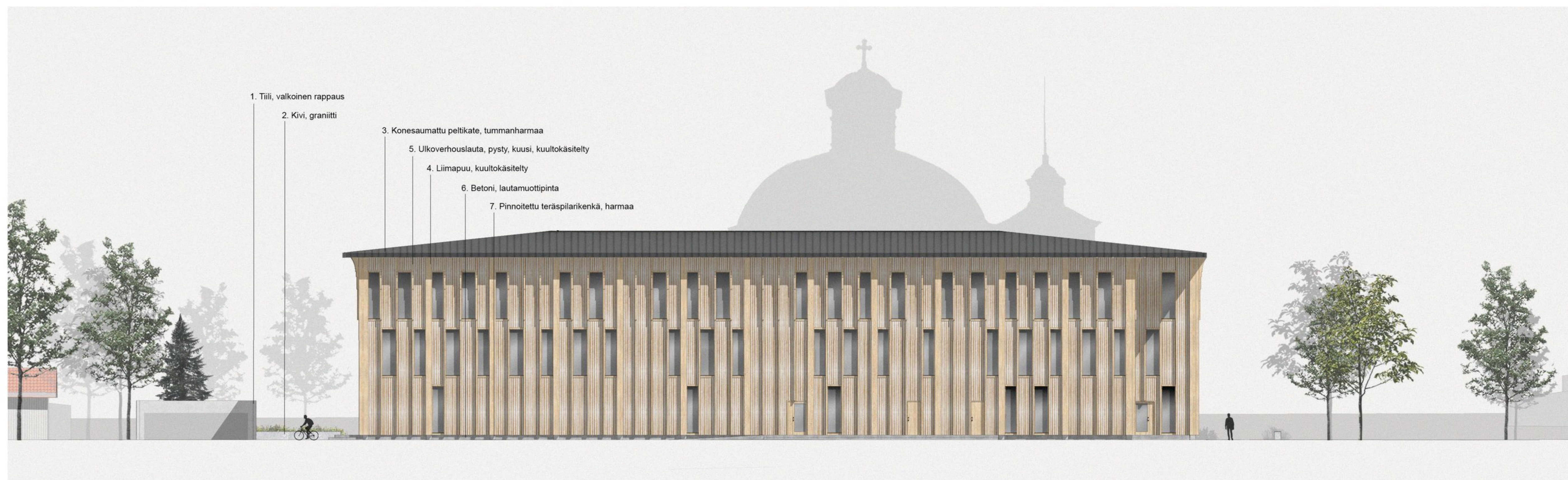
Julkisivu länteen 1:250
