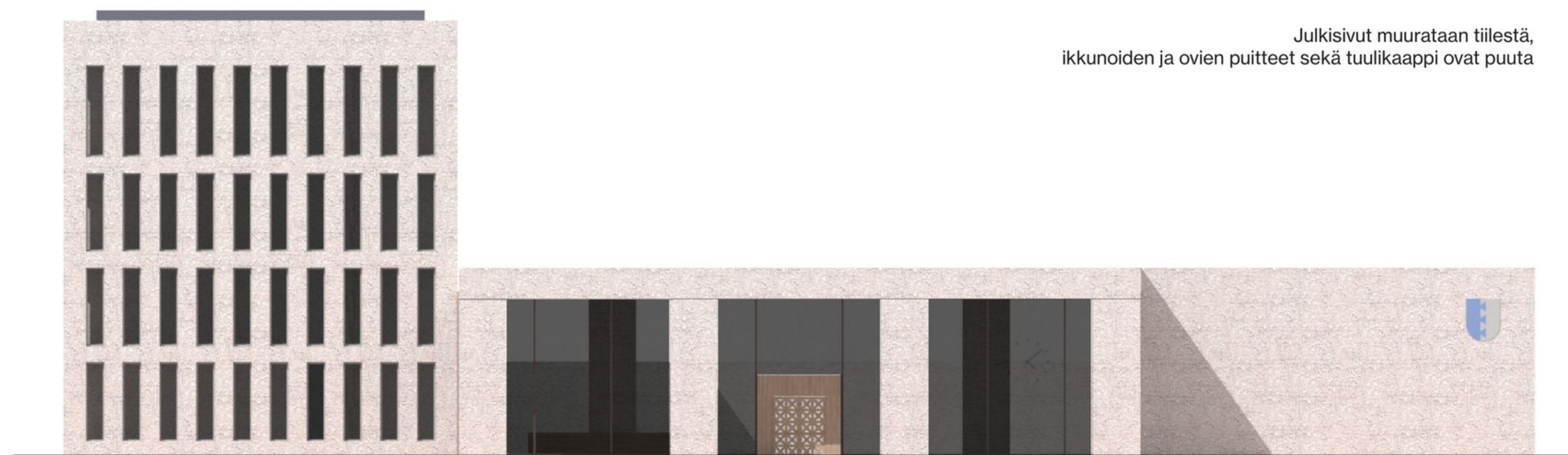
Julkisivu etelään 1:250
