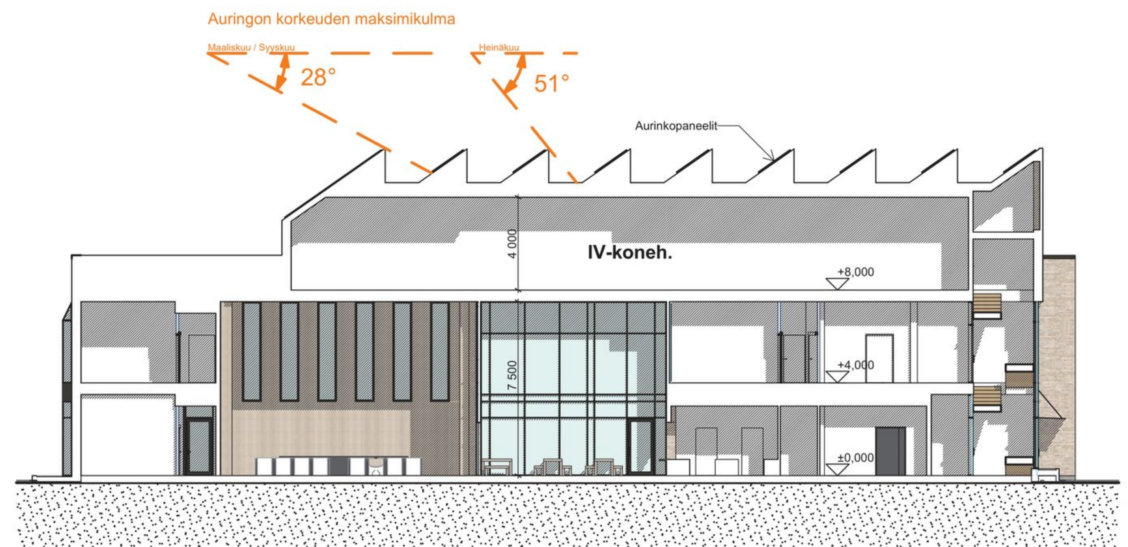
Leikkaus D-D
