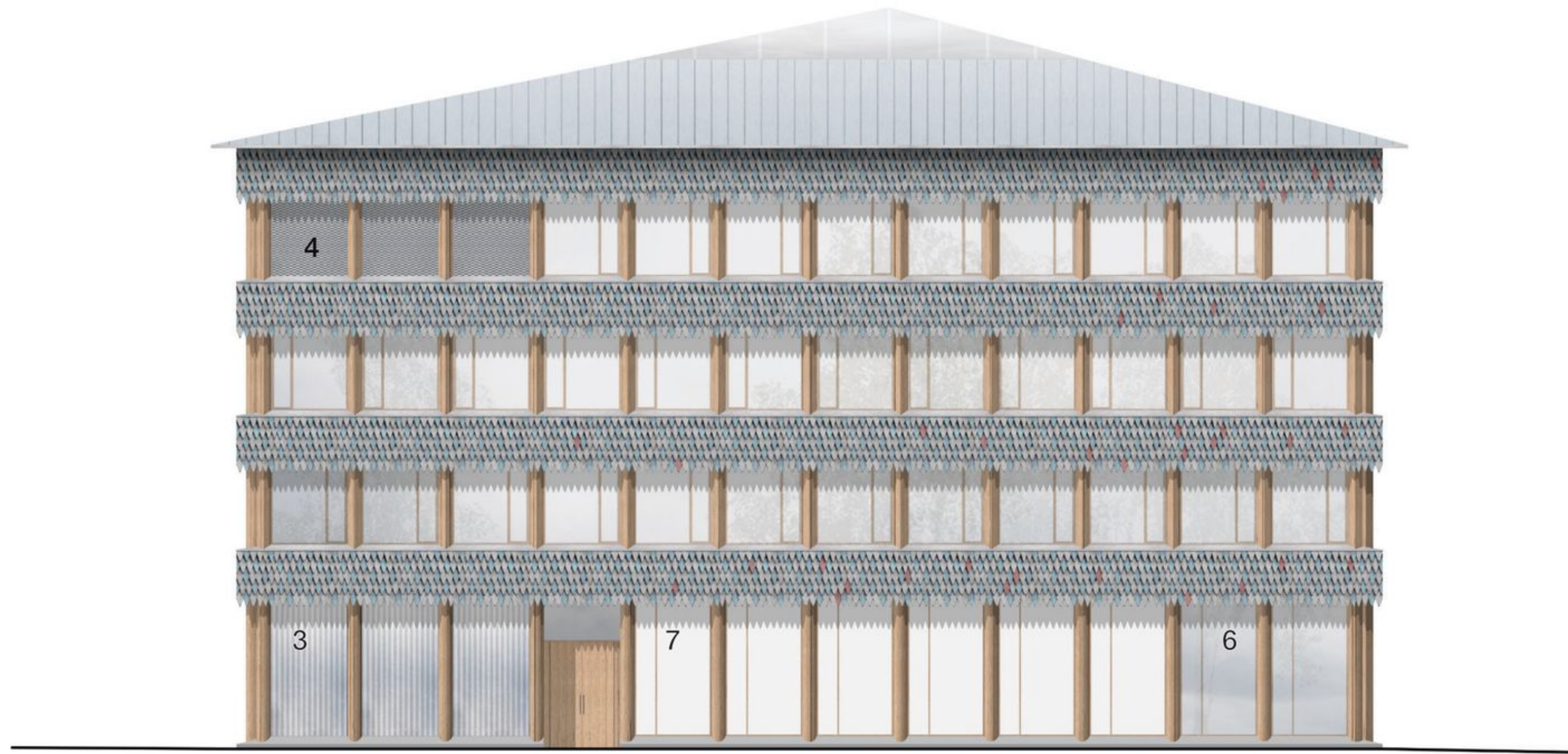
Julkisivu länteen 1:250
