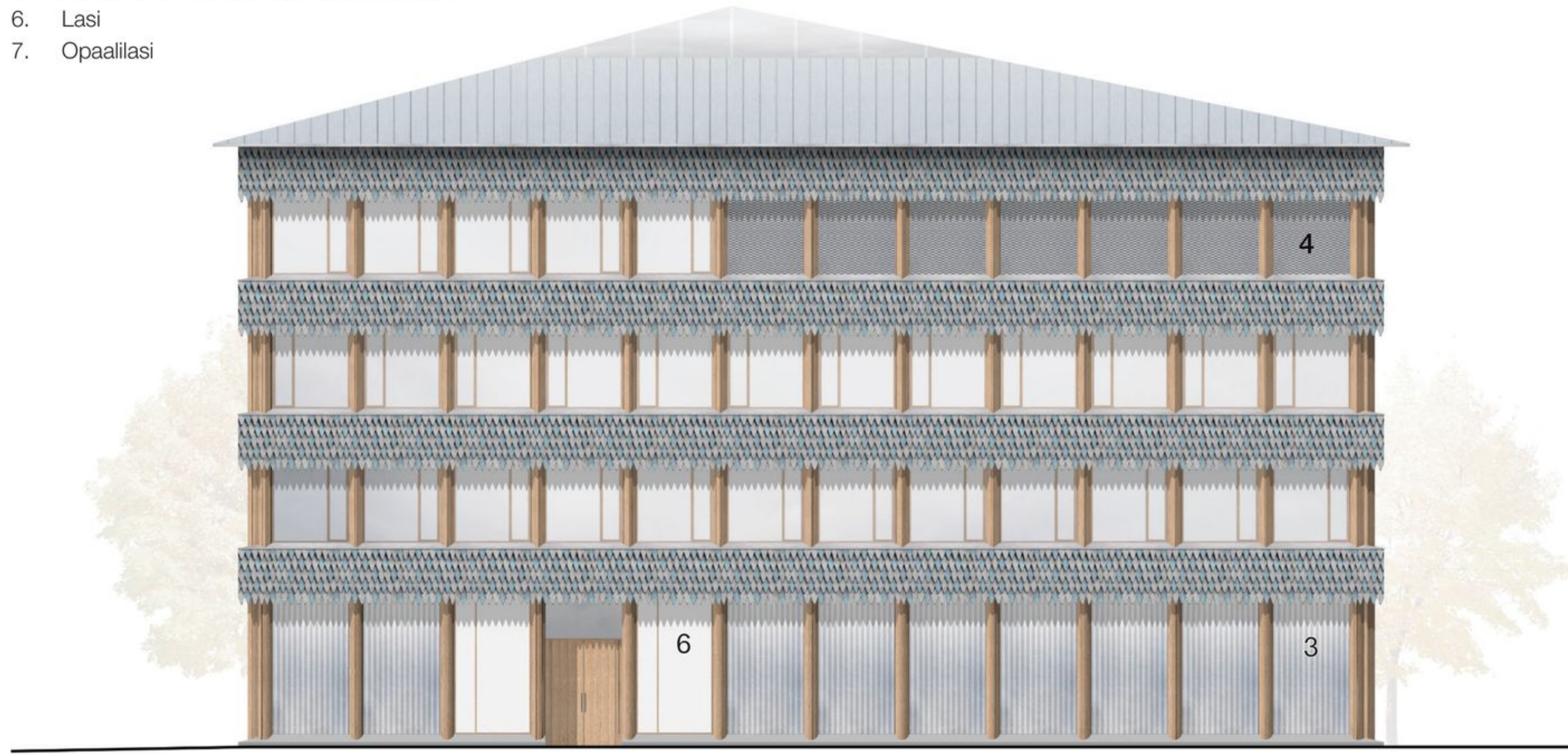
Julkisivu pohjoiseen 1:250
