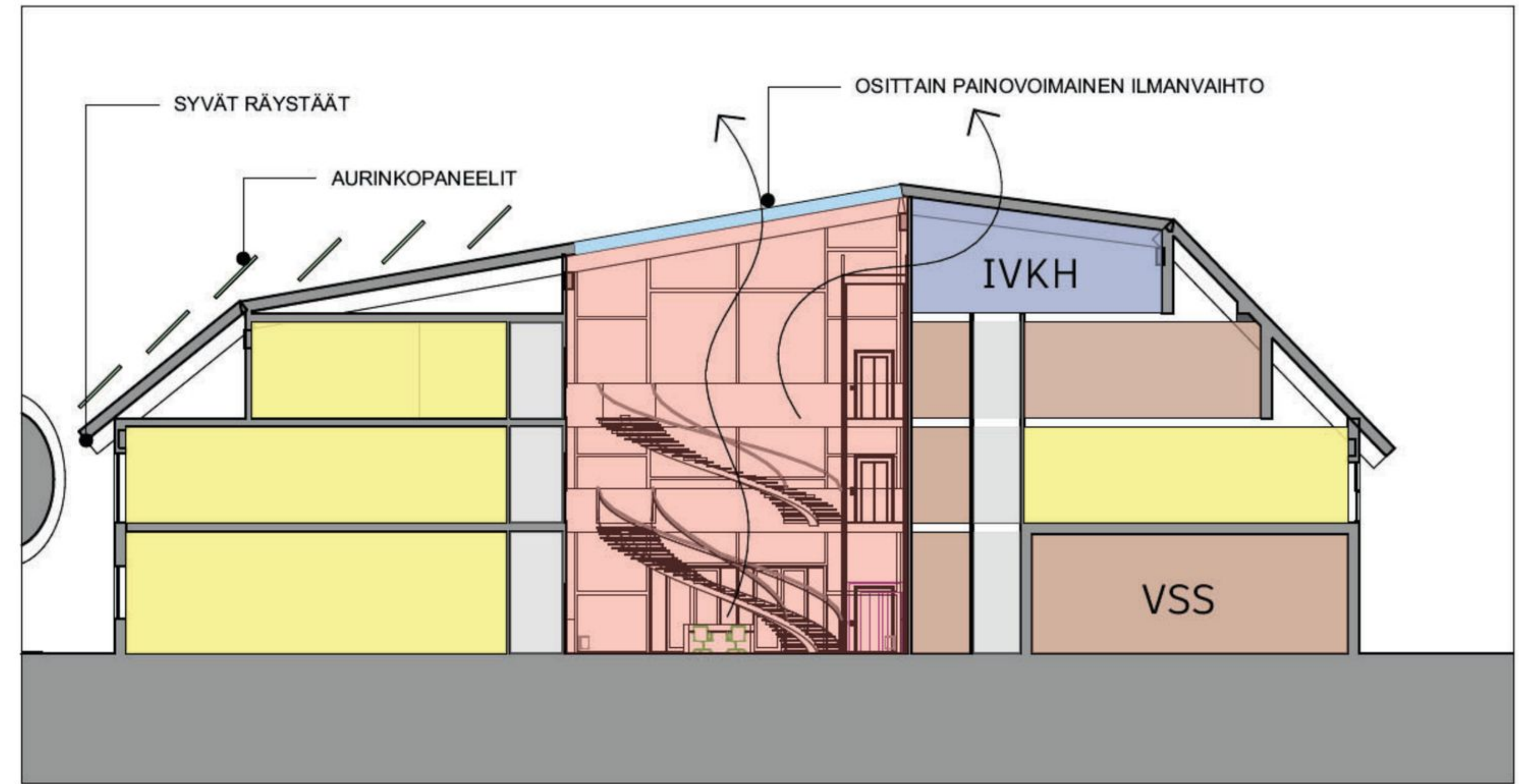
LEIKKAUS A-A
