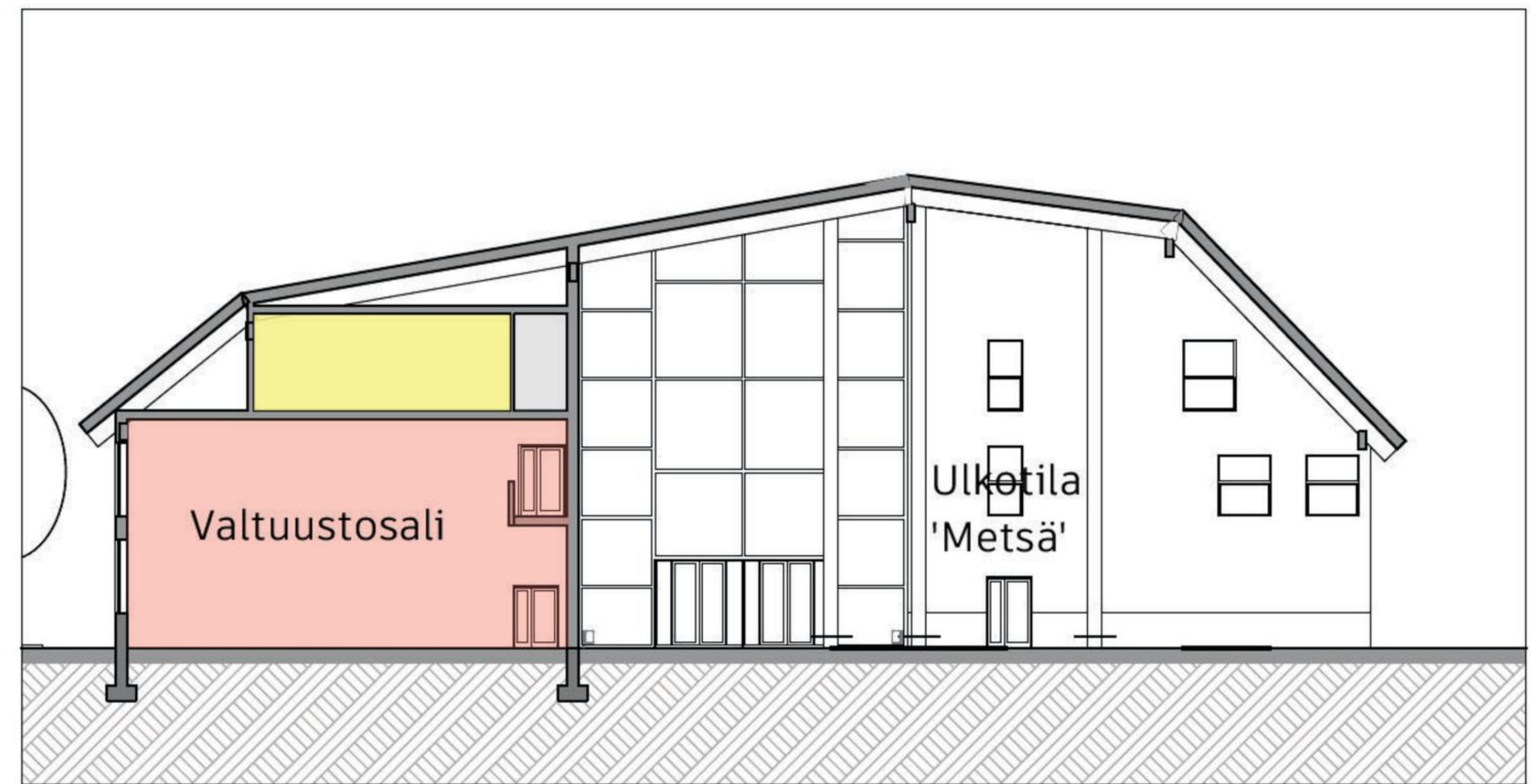
LEIKKAUS B-B
