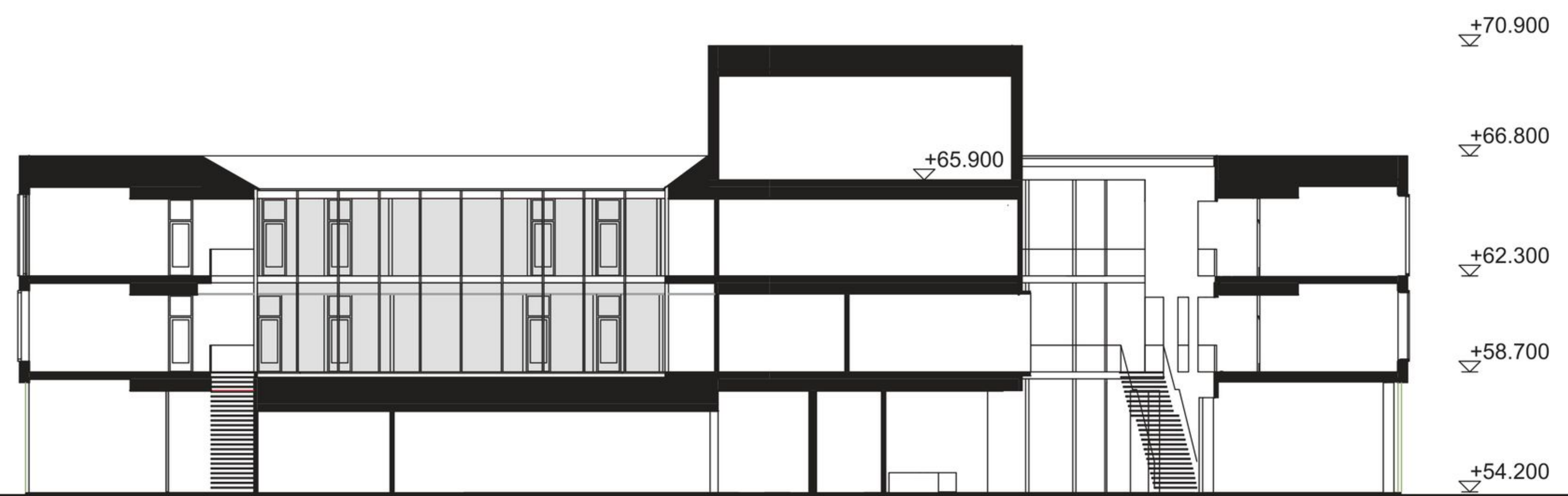
LEIKKAUS A-A
