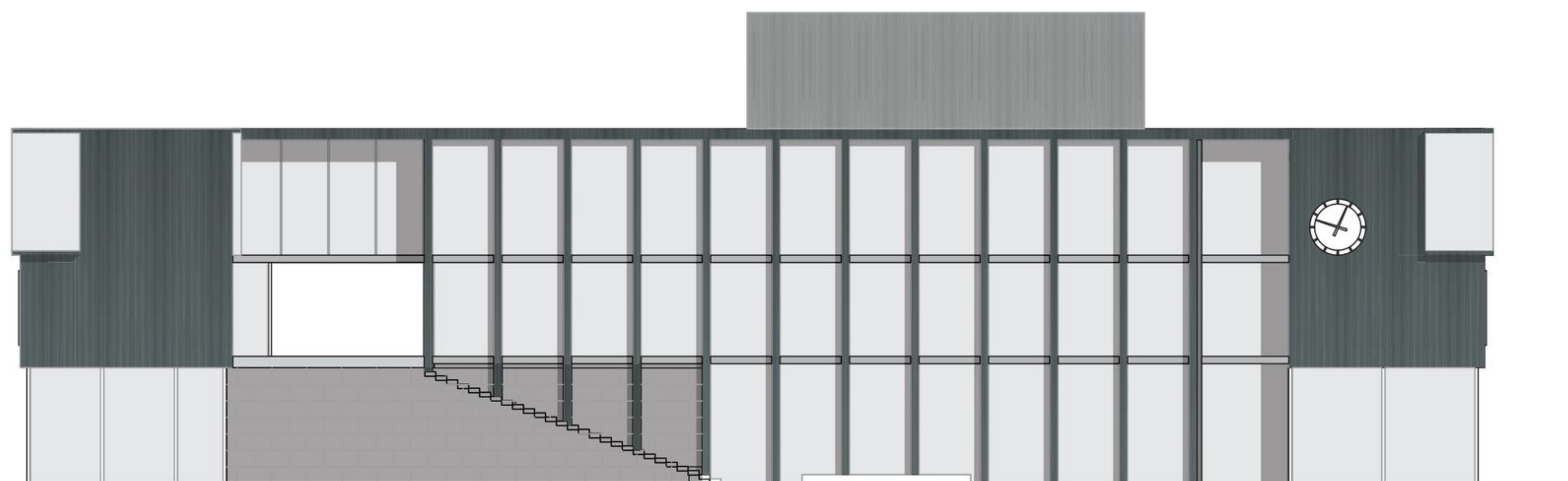
JULKISIVU ETELÄÄN
