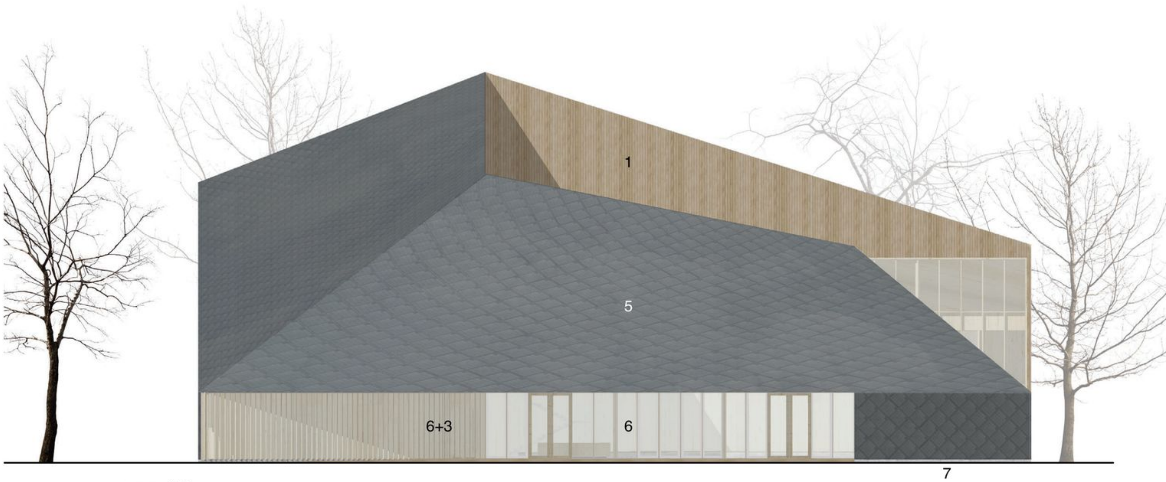
JULKISIVU ETELÄÄN 1:300
