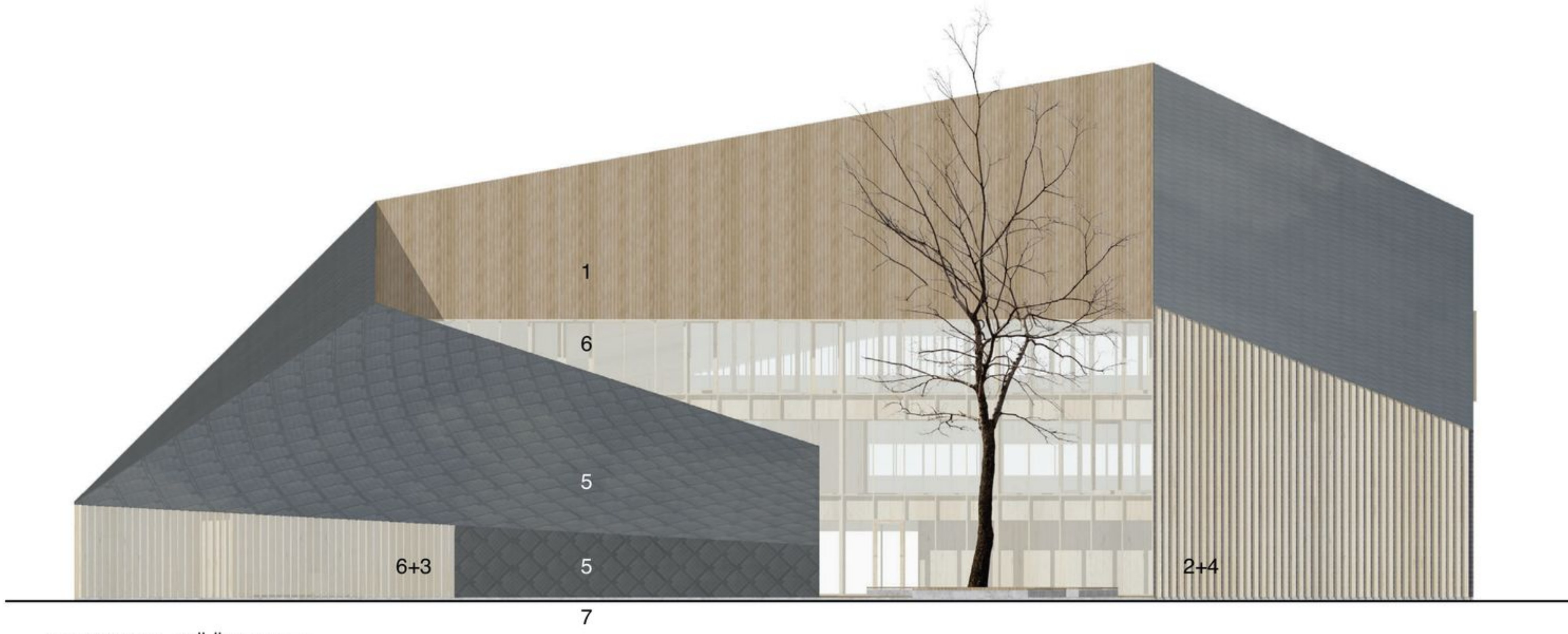
JULKISIVU ITÄÄN 1:300
