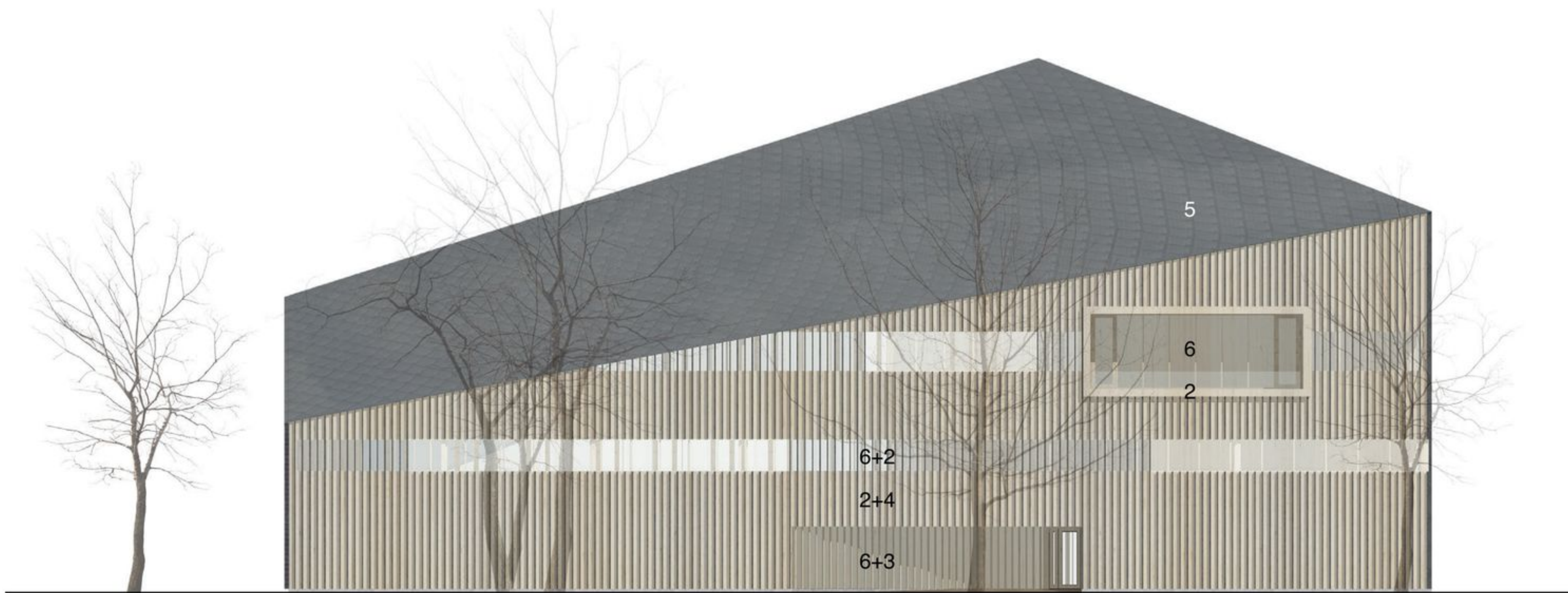
JULKISIVU POHJOISEEN 1:300
