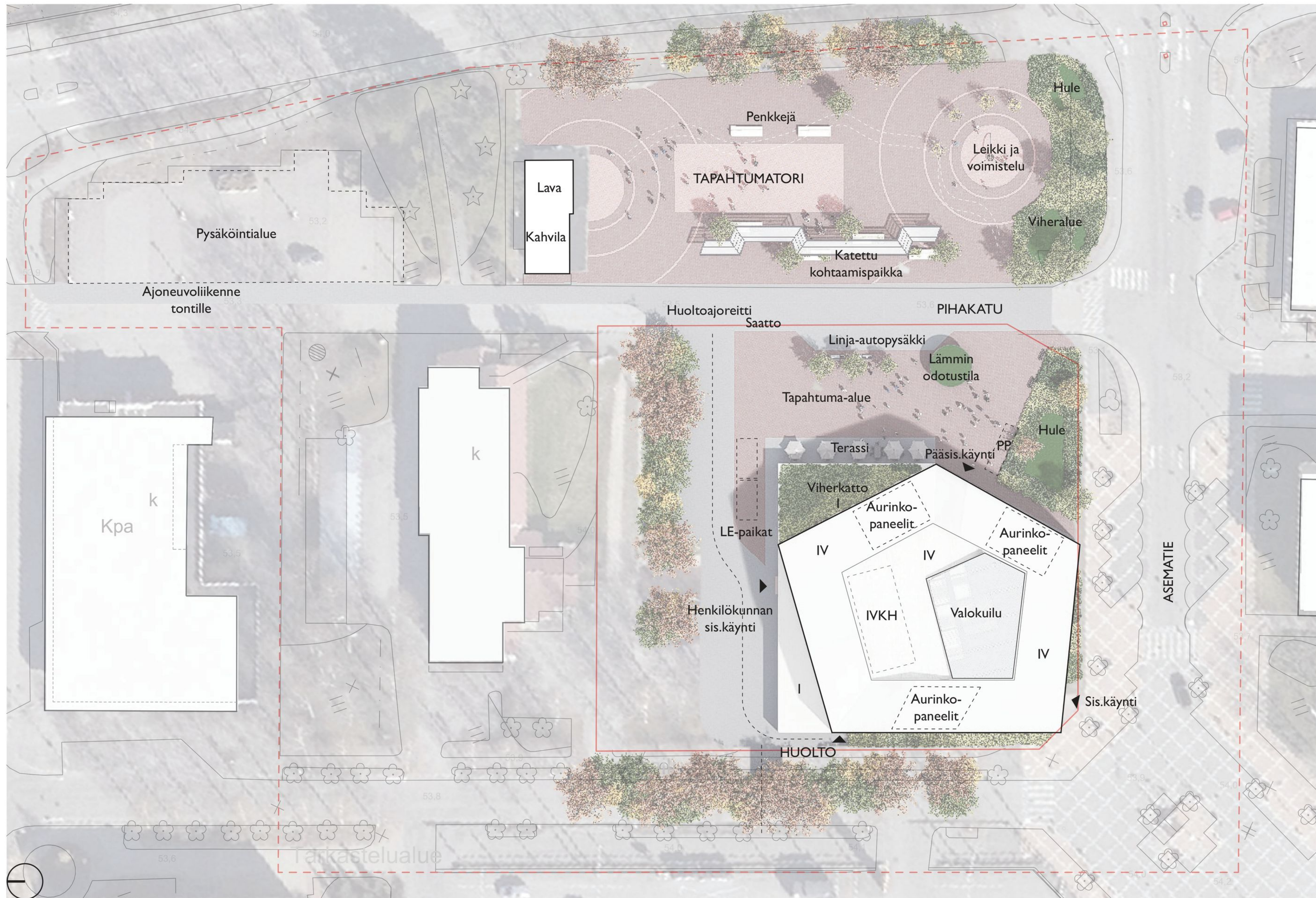
Asemapiirros 1:500 koko kilpailualueesta
