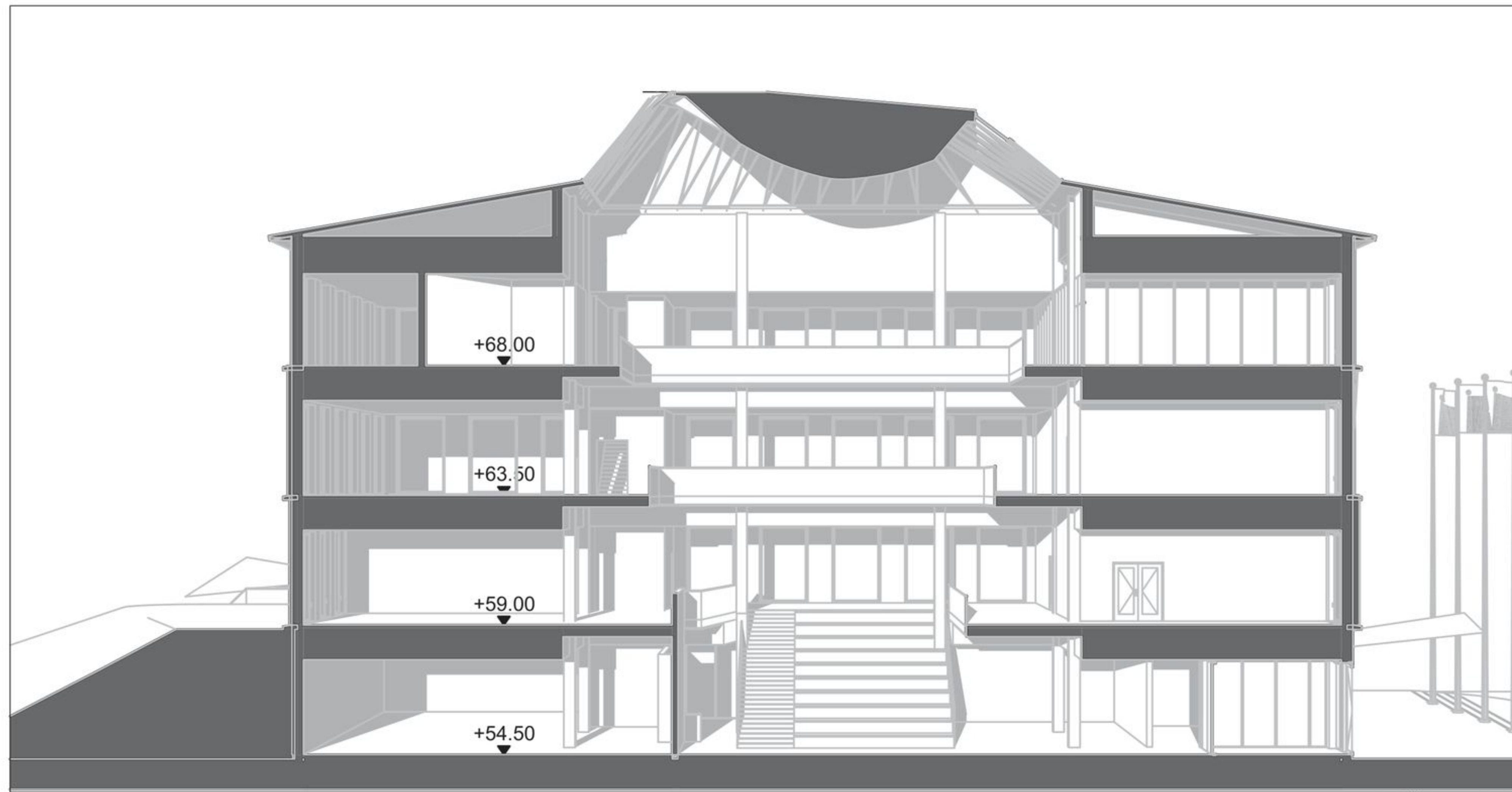
Leikkaus A-A
