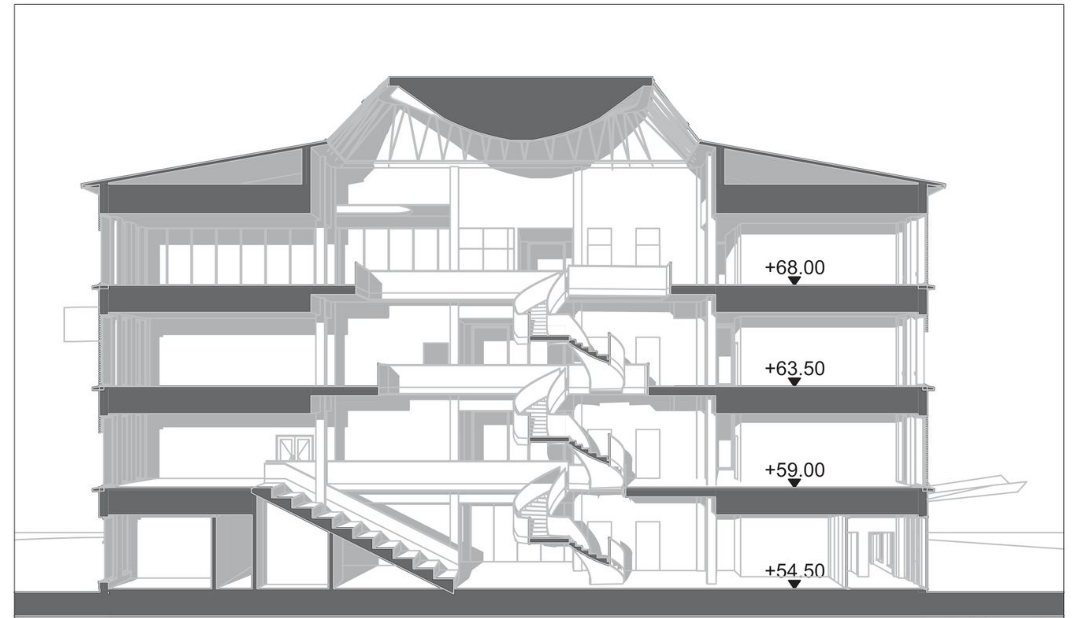
Leikkaus B-B
