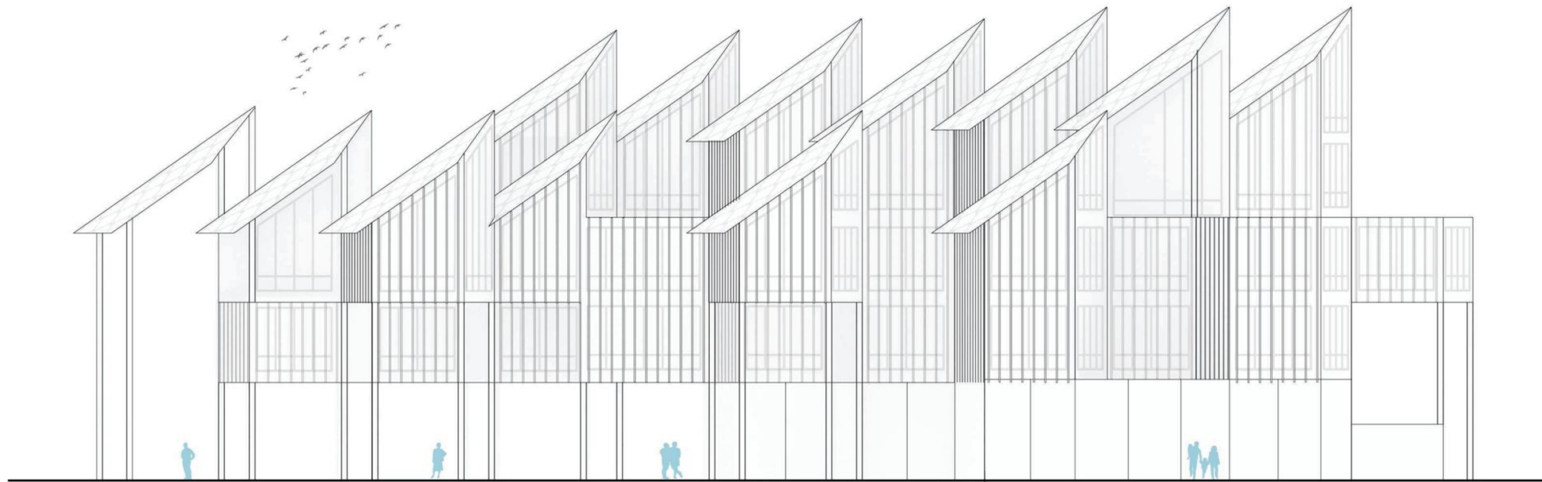
Julkisivu kaakkoon
