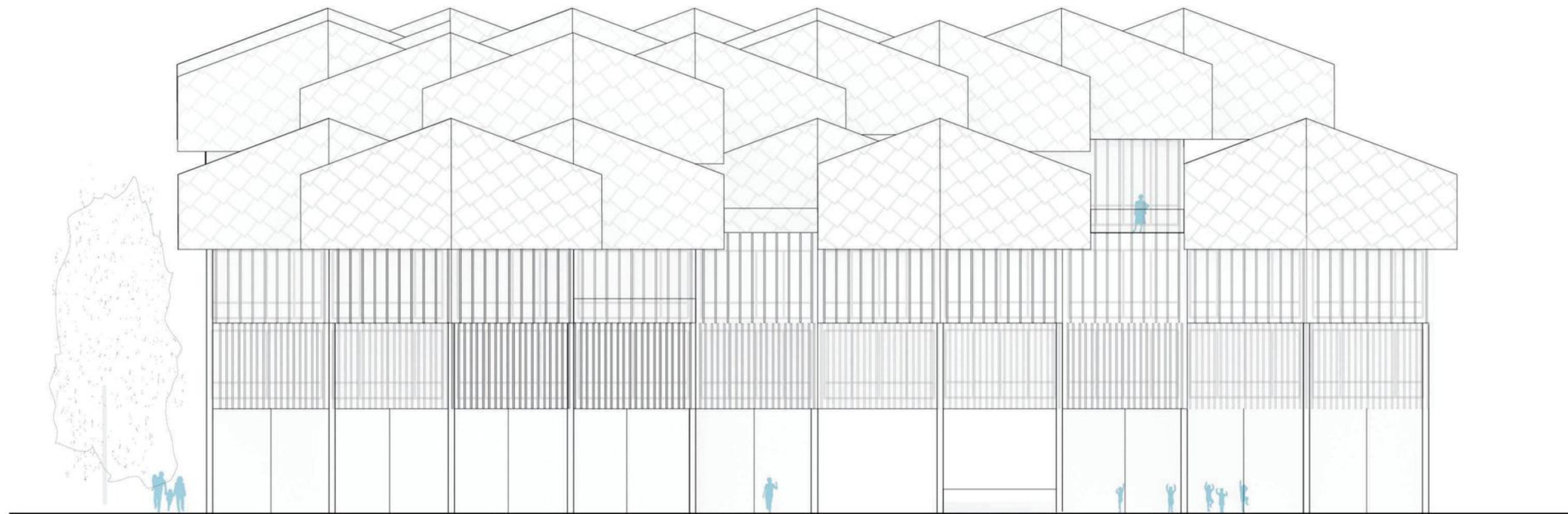
Julkisivu lounaiseen
