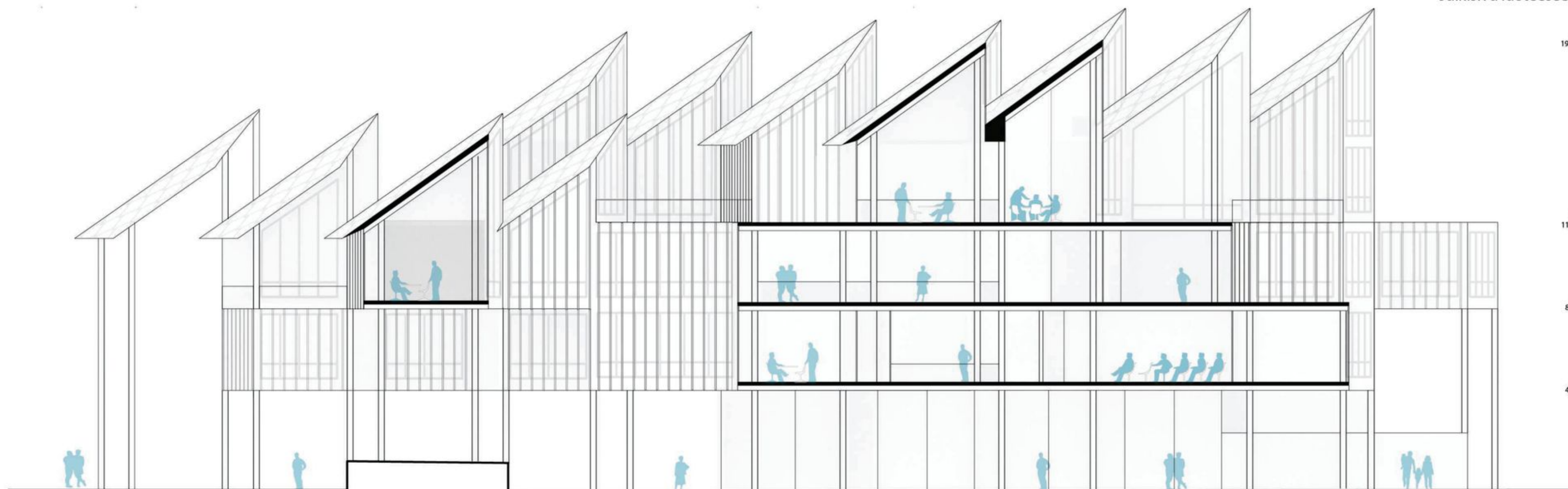
Leikkaus A-A
