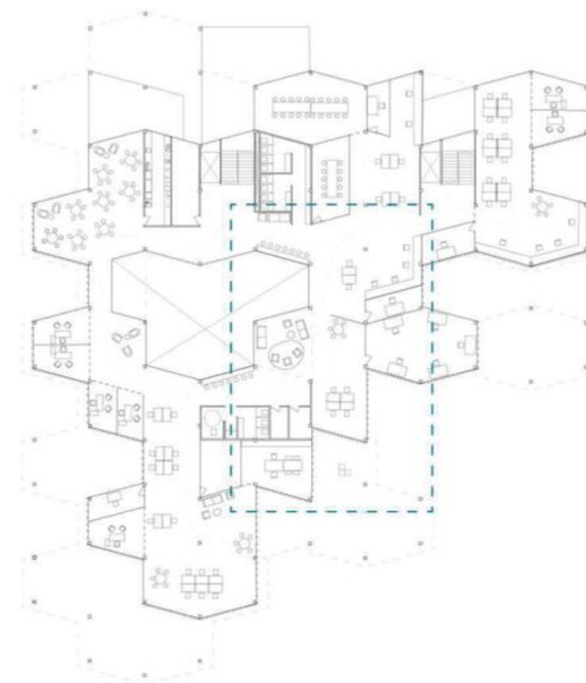
kerros 1
